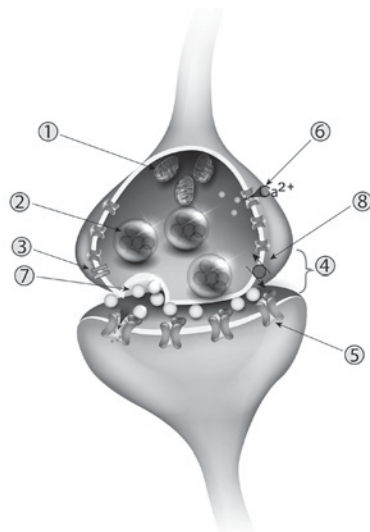
Abb. 7: Synapse schematisch
