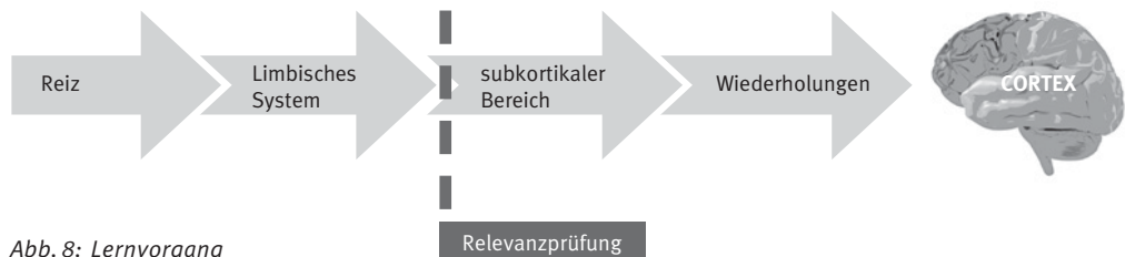
Abb. 8: Lernvorgang
